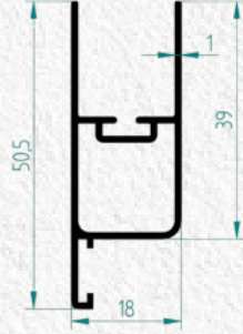
Ürün (SKU): 1203 Ağırlık (Weight): 413 gr / m. M3 PLİSE DIŞTAN TAKMA KASA P. M3 SLIM FS OUTSIDE MOUNTED FRAME
