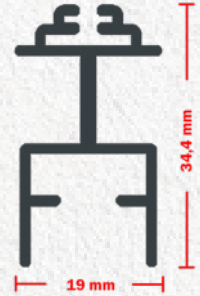
Ürün (SKU): 1253 Ağırlık (Weight): 284 gr / m. M2 18 MM PLİSE SİNEKLİK KANAT PROFİLİ M2 SLIM PLEATED FLY SCREEN SLIDING PROFILE
