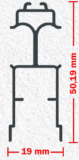
Ürün (SKU): 1212 Ağırlık (Weight): 358 gr / m. 18 MM PLİSE SİNEKLİK KANAT PROFİLİ SLIM PLEATED FLY SCREEN SLIDING PROFILE
