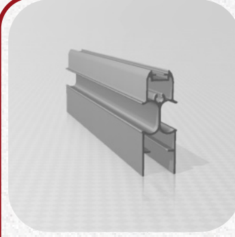
Ürün (SKU): 1202 Ağırlık (Weight): 503 gr / m. M3 18 MM PLİSE KANAT PROFİLİ M3 SLIM PLEATED FLY SCREEN SLIDING PROFILE
