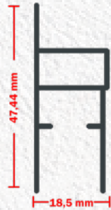
Ürün (SKU): 1210 Ağırlık (Weight): 267 gr / m. 18 MM PLİSE SİNEKLİK İÇTEN TAKMA KASA PROFİLİ SLIM PLEATED FS INSIDE MOUNTED FRAME PROFILE
