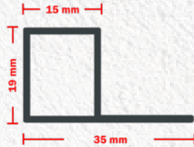
Ürün (SKU): 1340 Ağırlık (Weight): 234 gr / m. İÇE AÇILIM P PROFİLİ P PROFILE FOR HINGED FS OPENS INSIDE
