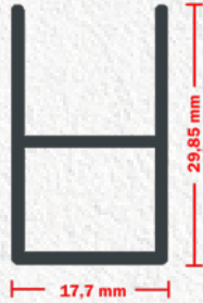
Ürün (SKU): 1252 Ağırlık (Weight): 217 gr / m. M2 18 MM PLİSE SİNEKLİK KASA PROFİLİ M2 SLIM PLEATED FLY SCREEN FRAME PROFILE
