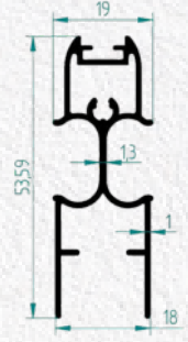
Ürün (SKU): 1202 Ağırlık (Weight): 503 gr / m. M3 18 MM PLİSE KANAT PROFİLİ M3 SLIM PLEATED FLY SCREEN SLIDING PROFILE
