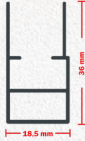
Ürün (SKU): 1211 Ağırlık (Weight): 258 gr / m. 18 MM PLİSE SİNEKLİK KASA PROFİLİ SLIM PLEATED FLY SCREEN FRAME PROFILE
