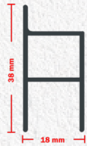
Ürün (SKU): 1250 Ağırlık (Weight): 265 gr / m. M2 PLİSE SİNEKLİK İÇTEN TAKMA KASA PROFİLİ M2 SLIM PLEATED FS INSIDE MOUNTED FRAME PROFILE
