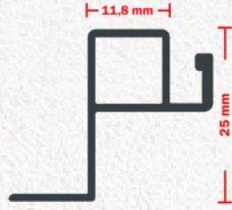
Ürün (SKU): 1310 Ağırlık (Weight): 250 gr / m. İÇTEN TAKMA SİNEKLİK PROFİLİ PRACTICAL FLY SCREEN PROFILE (INSIDE MOUNTED)
