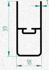
Ürün (SKU): 1201 Ağırlık (Weight): 360 gr / m. M3 18 MM PLİSE KASA PROFİLİ M3 SLIM PLEATED FLY SCREEN FRAME PROFILE
